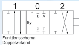
Walvoil SD5/2 Funktion: 1x doppelwirkend 1x einfachwirkend
