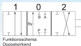
Walvoil SD5/2 Funktion: 1x doppelwirkend 1x doppelwirkend mit Schwimmstellung
